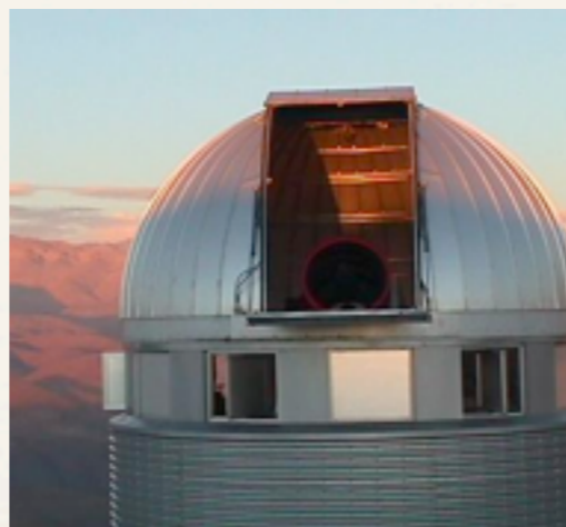
CORALIE
