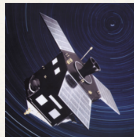
HIPPARCOS
